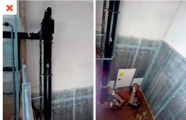
Le système d'alimentation entre le silo enterré et la chaudière est composé de 5 vis sans fin. Les deux premières (1 et 2), horizontales, permettent l'acheminement du combustible vers la chaufferie. Les trois autres (3, 4 et 5) servent à l'acheminement vers le foyer. ©AQC
