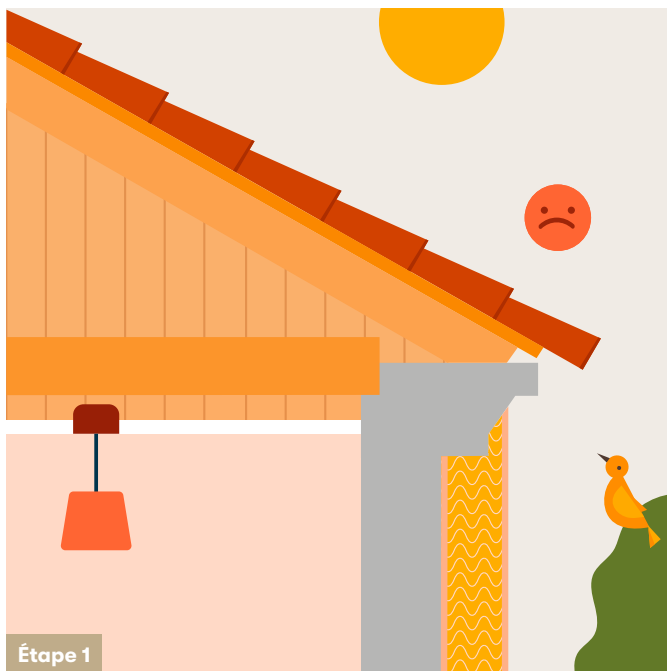
Isolation des murs par l'extérieur avec débord de toit maçonné
