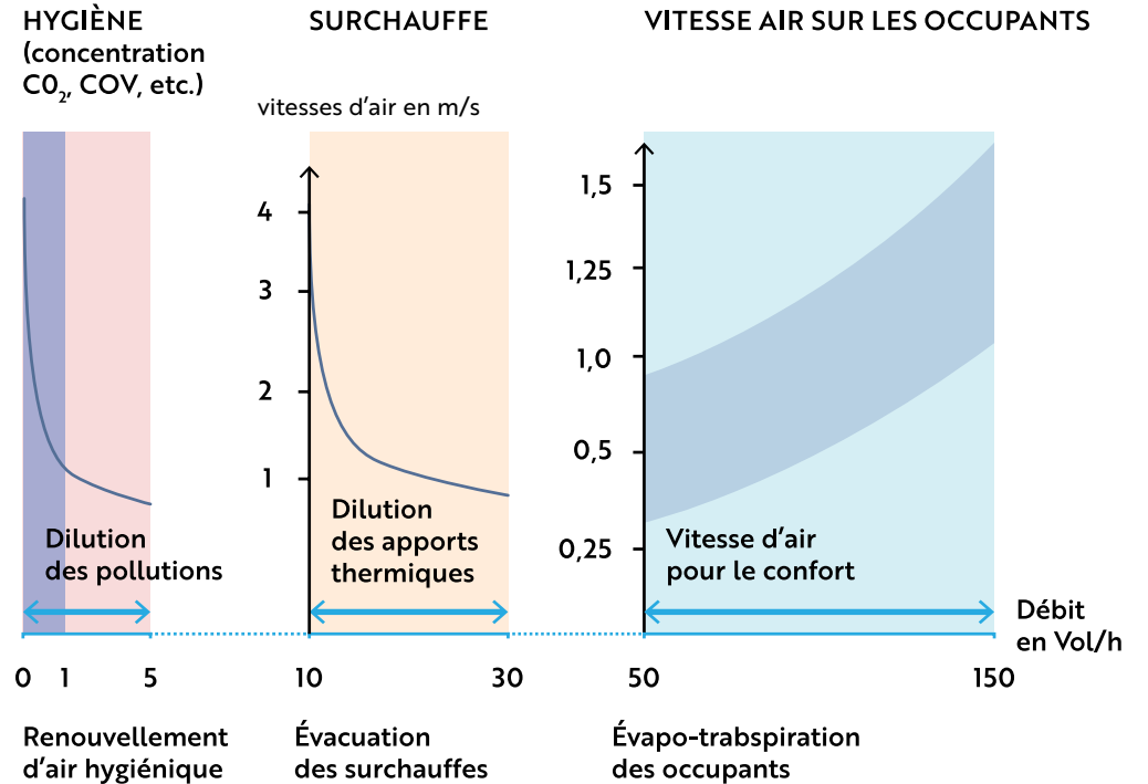
Les 3 régimes de ventilation des bâtiments
