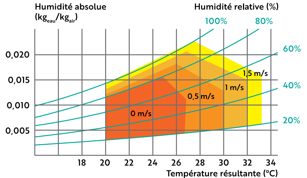
Diagramme de Givoni
